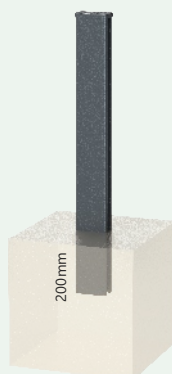
POTEAU 76x41 à sceller direct Hauteur maxi conseillée 1.600mm
