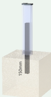
POTEAU 76x41 à sceller avec tube 30x30 acier Longueur 500mm Hauteur maxi conseillée 1.100mm
